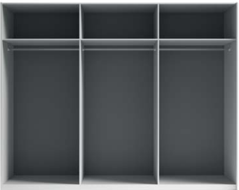
KORPUS SZAFY 270 TYP 59 →/↑/↗ 270/211/60 cm
